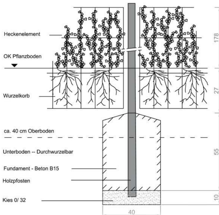
Fundament Holzpfosten
